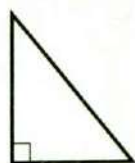
Прямоугольный треугольник
