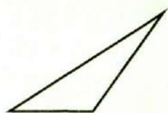
Тупоугольный треугольник
