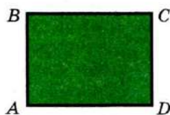
Прямоугольник ABCD
